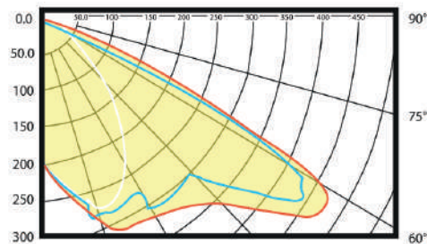
ARRO 1 250W HPSV
